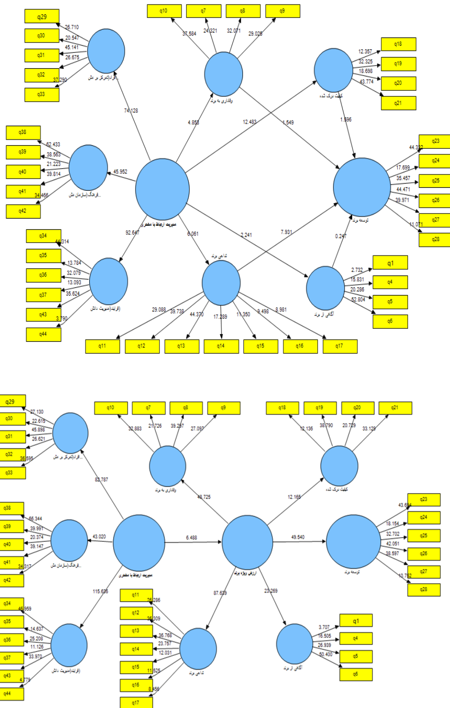
تصویر ۴- مدل ساختاری در حالت اعداد معناداری (t-value) برای مدل فرعی و اصلی پژوهش (پژوهشگر)
