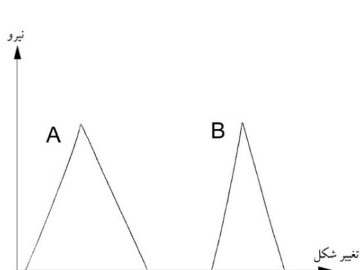
شکل ۲: منحنی نیرو - تغییر شکل برای دو فنر با سختی کم (A) و زیاد (B)
